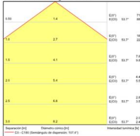
Emisión de luz 1 / Diagrama conico
